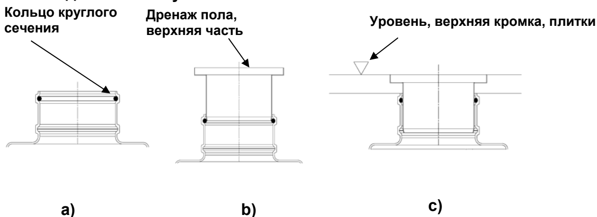
Рис. 6 Удаление заглушки
